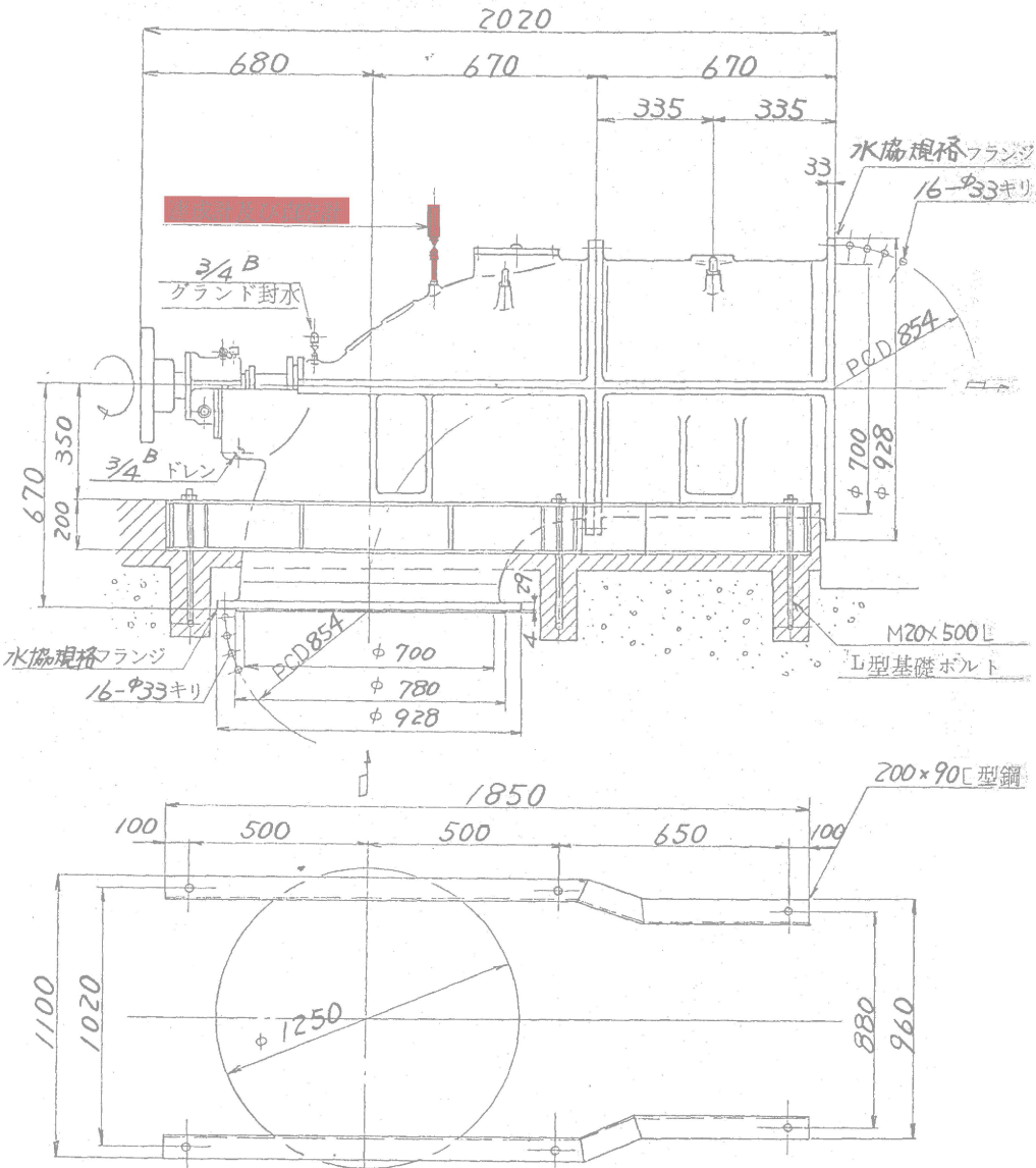
ベース平面図
